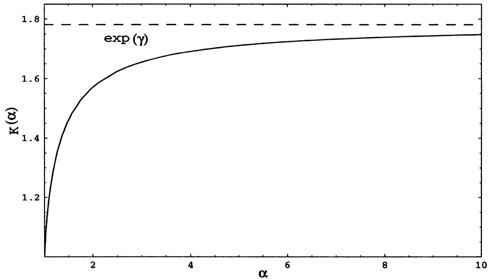
FIG. 1. Function K(\alpha) .
